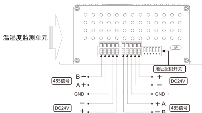
温湿度监测单元端子接线定义图
