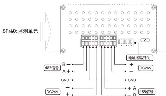
SF6&氧气监测单元端子接线定义图
